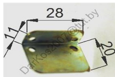
Фиксатор мебельный №18
