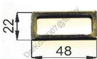
Рамка №10
