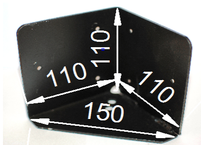
Уголок
