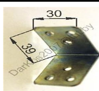
Уголок УШ-4-1 №15
