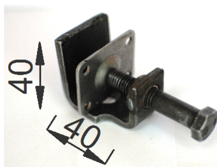
струбцина
