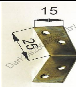
Уголок мебельный 15x25 №2
