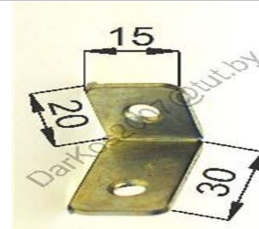
Уголок УШ-4-1 №15
