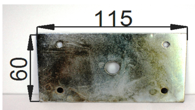
Пластина 60x115
