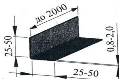
Уголок №8
