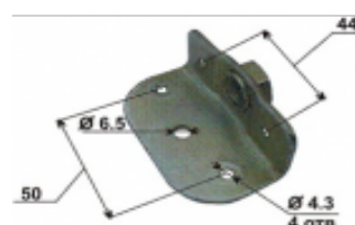
Уголок для крепления опоры колесной
