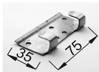
Уголок для крепления опоры колесной
