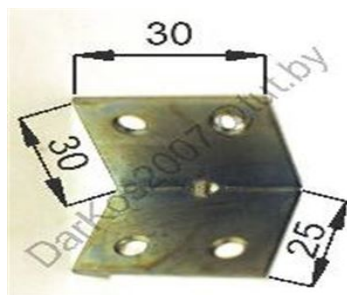
Уголок 25x30x1,2 с ребром жесткости №28
