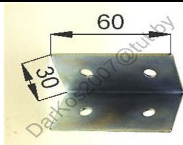
Уголок мебельный 30x60 №4
