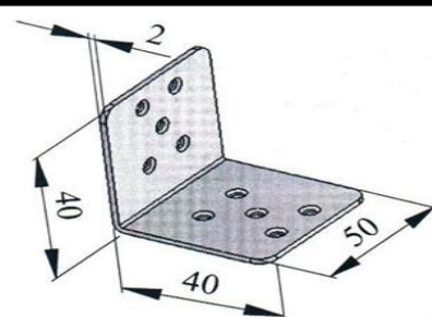
Уголок 40x40x50 №23
