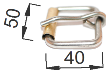
Застежка
