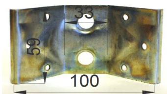
Опора угловая(обойма) №7
