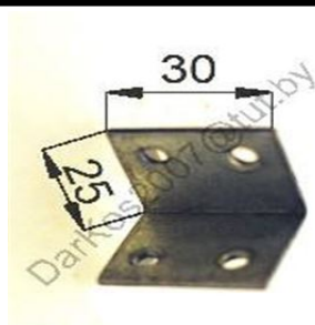
Уголок ФБ 0080 25x30 №14
